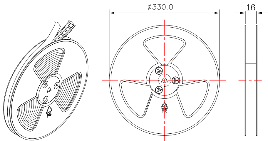
1 Reel : 2500PCS
