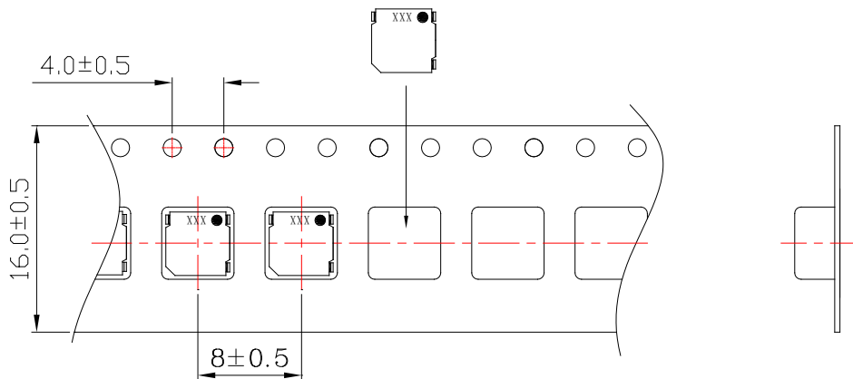
1 Reel : 2500PCS
